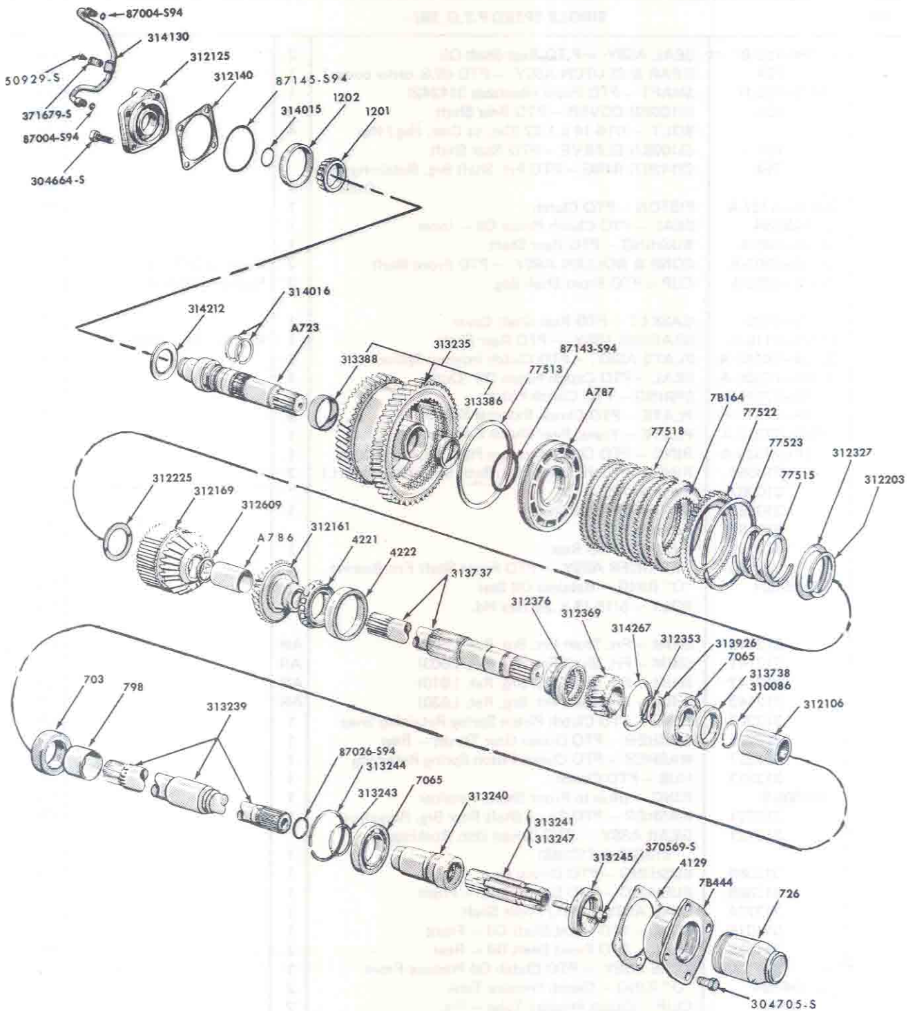
FIG. 7D8 2 SPEED P.T.O. 59/-
