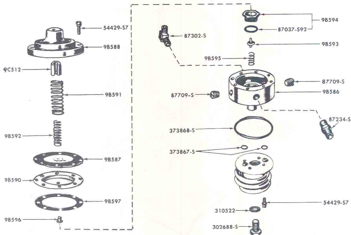
FIG. 9E2 - L.P.G. VAPORIZOR ASSY. - 1961/
