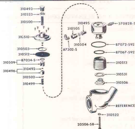
FIG. 9E1 - L.P.G. VAPORIZER & RELATED PARTS 57/60
